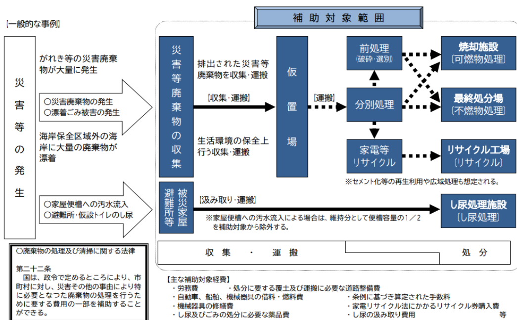
図2-18 災害等廃棄物処理事業の業務フローと補助対象範囲
